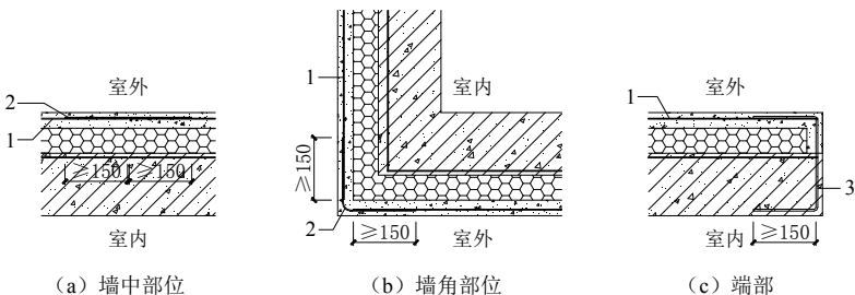
图 5.2.8 防护层附加镀锌电焊网
