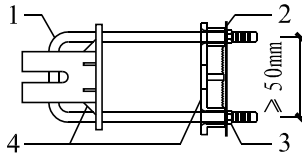
图 4.1.6 U形连接件
